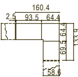
Angolo con 1 ante scorrevole da cm 96 e 1 ante scorrevole da cm 72. Corner with a 72 cms + a 96 cms sliding door.
