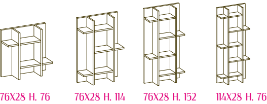
Pannelli orizzontali/verticali profondità 28 cm. con mensole legno (sp. 4) vetro (sp. 0,8) Horizontal/vertical panels D. 28 cms with wood shelves (Th. 4) glass (Th. 0.8)
